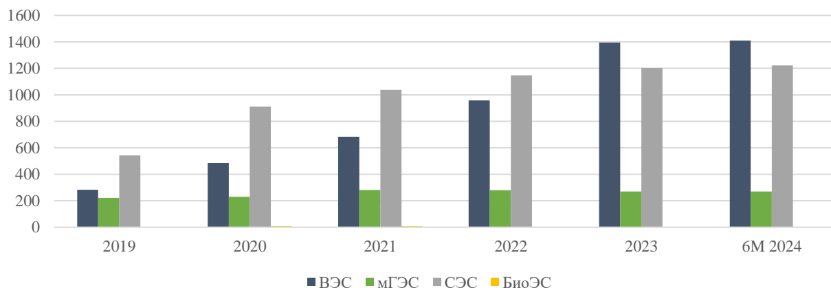
Установленная мощность станций ВИЭ в РК, МВт
