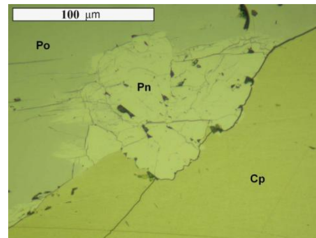
Фото. Минералогическое описание шлифа. Зерна пентландита (Pn) локализованы между пирротином (Po) и халькопиритом (Cp).
