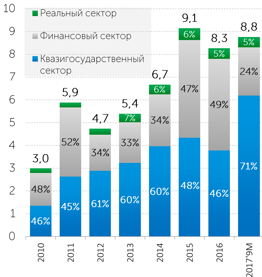
Структура капитализации рынка корпоративных облигаций в разрезе основных секторов экономики
