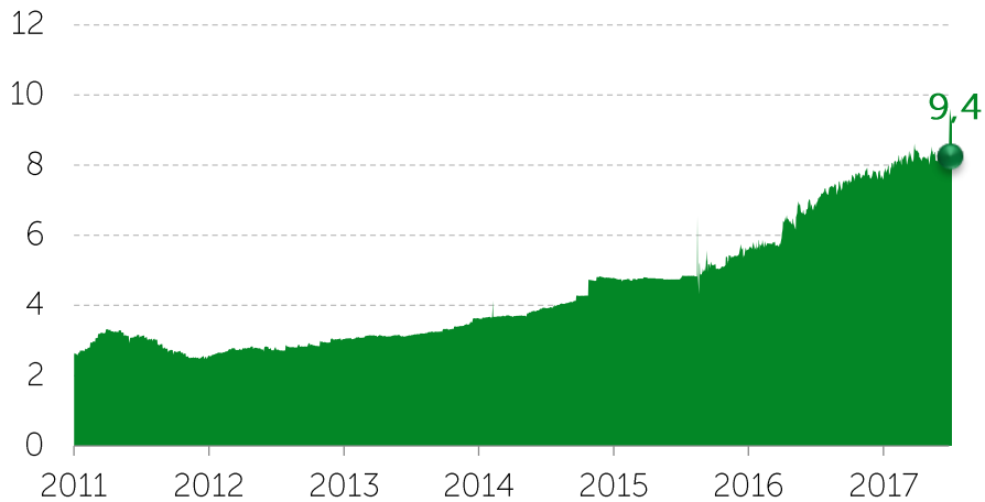
Сумма государственного долга, трлн KZT
